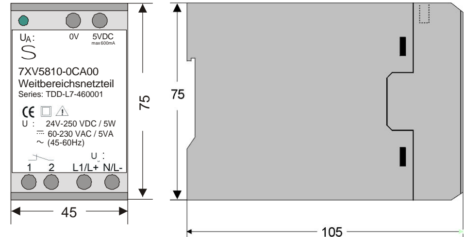
Abb. 4: Maßbilder
