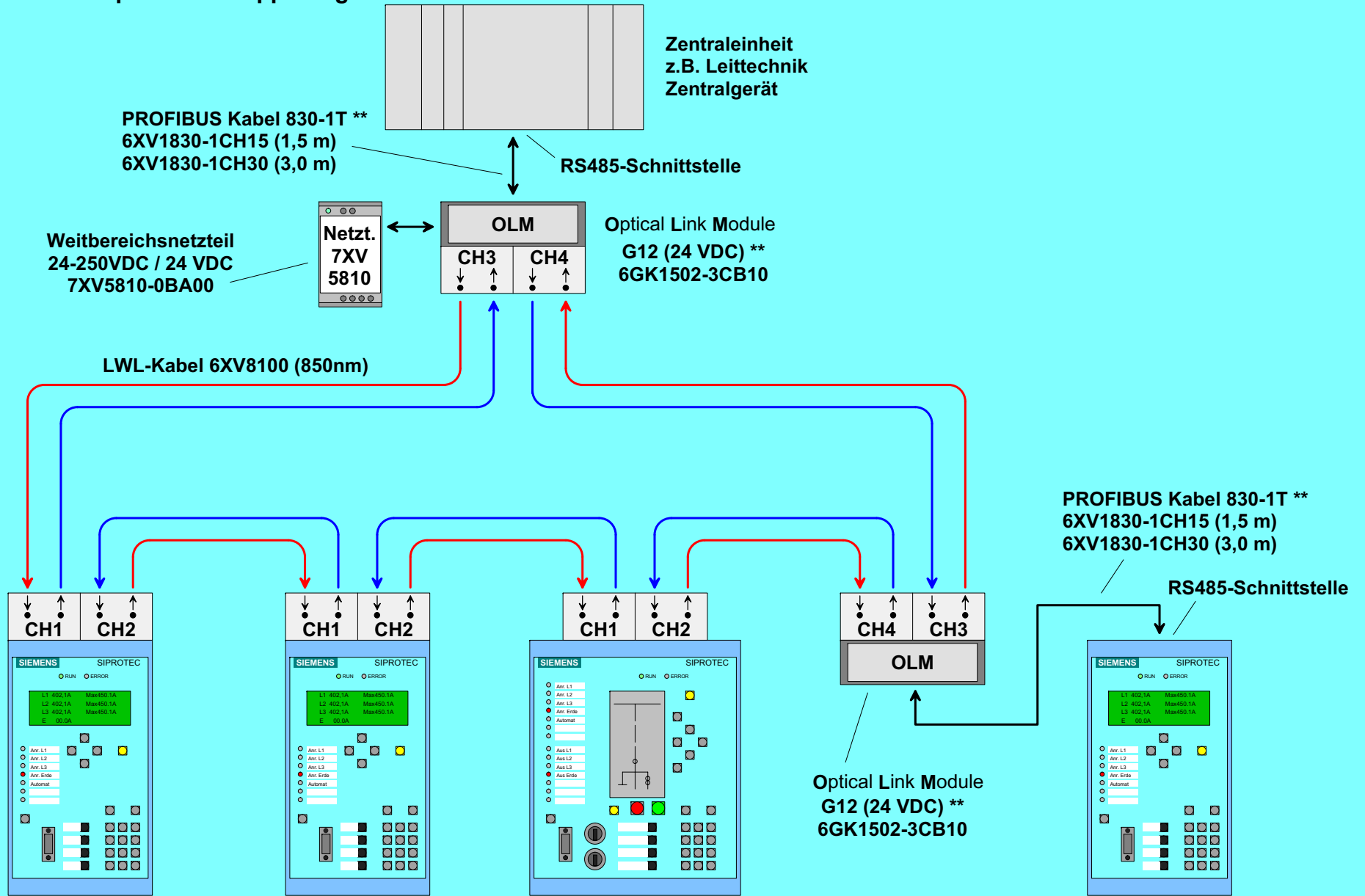
SIPROTEC 4 Schutzgerät mit RS485 PROFIBUS Schnittstelle
