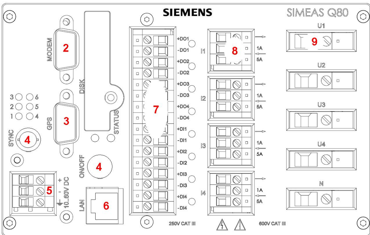
SIMEAS Q80 7KG8080 - 0 mit 4 Spannungs und 4 Stromeingängen
