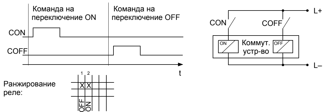
Рис. В-5 1-полюсная двойная команда
