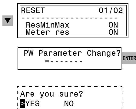
Рис. 6-28 Сброс счетно-импульсных величин и минимальных/максимальных значений
