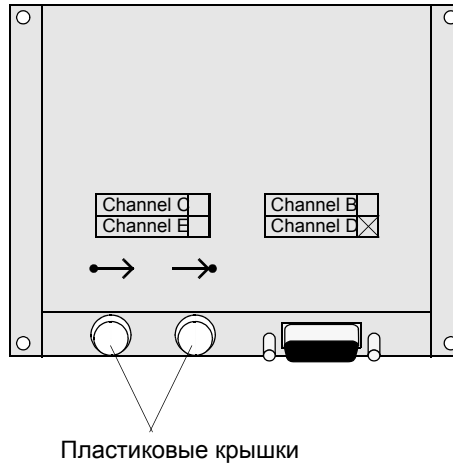
Рис. 2-34 Корпус с 9-контактным миниатюрным разъемом D типа "мама"
