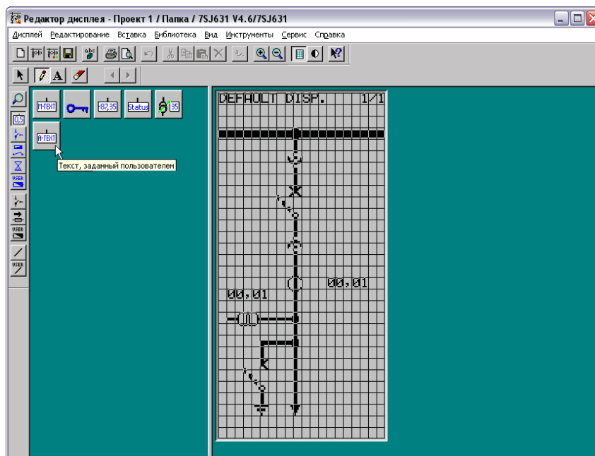
Рис. 5-52 Размещение пользовательского текста
