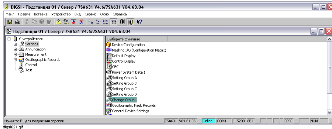
Рис. 6-40 DIGSI® 4 Опция переключения группы уставок
