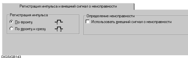
Рис. 5-21 Пример закладки Регистрация импульса и внешний сигнал неисправности
