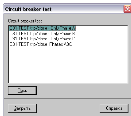
Рис. 6-49 DIGSI® 4 Проверка выключателя, пример
