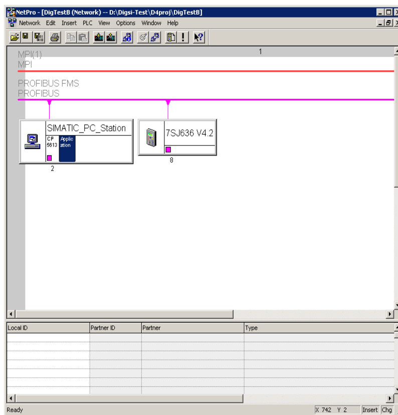
Рис. 7-58 NetPro с таблицей для конфигурирования устройств SIPROTEC
