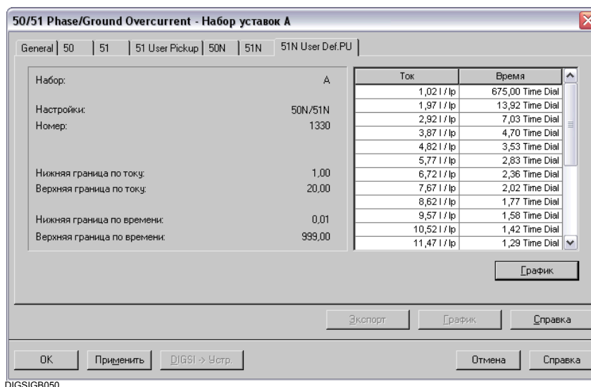
Рис. 5-84 Установка значений для табличных параметров
