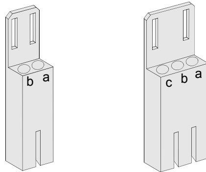
Рис. 2-26 2 и 3 контактный корпус разъема
