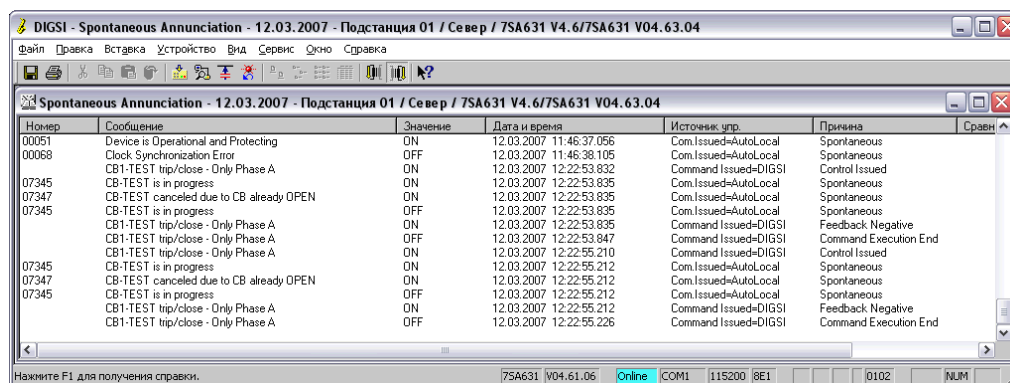
Рис. 6-50 DIGSI® 4 Спонтанные сообщения проверки выключателя, пример
