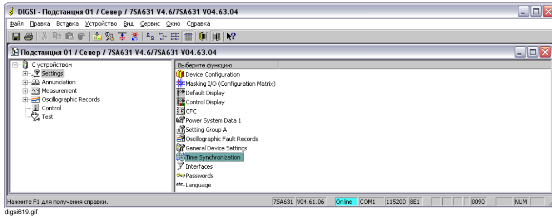
Рис. 6-37 DIGSI® 4 Выбор синхронизации времени
