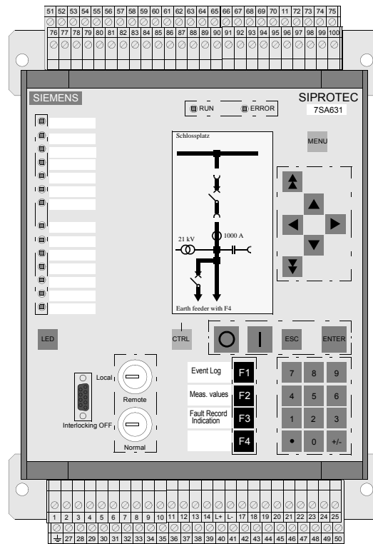
Рис. 2-12 Графический дисплей, размер корпуса 1/2 , пример устройства для наружной установки на панели без оптоволоконного соединения
