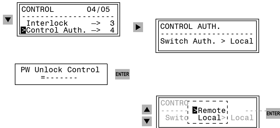
Рис. 6-62 Рабочее меню дисплея для разрешения на переключение (пример в режиме без блокировки)
