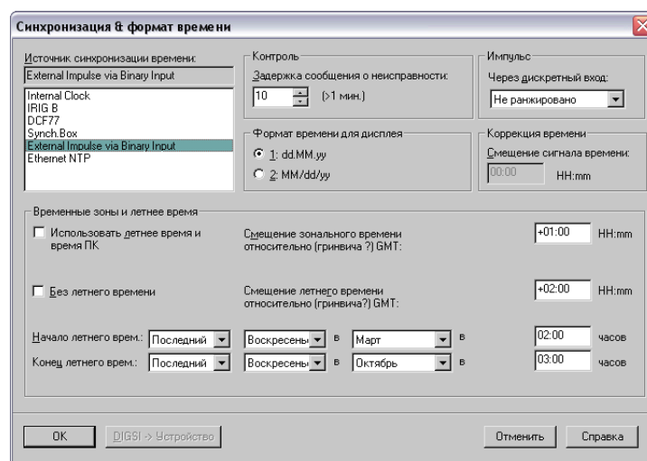
Рис. 5-77 Синхронизация и формат времени
