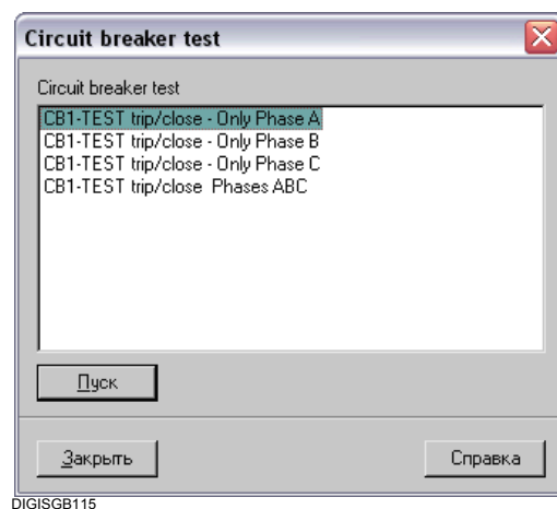
Рис. 8-5 Проверка выключателя
