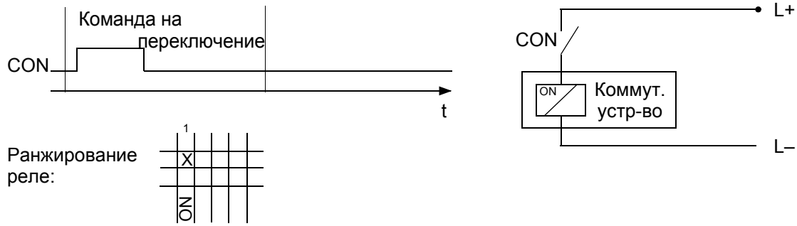
Рис. В-4 1-полюсная простая команда
