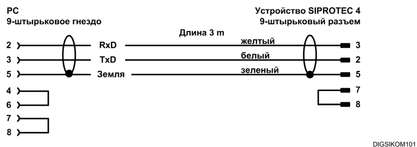
Рис. A-6 Электрическая схема для кабеля 7XV5100-4 между модемом и устройством SIPROTEC 4
