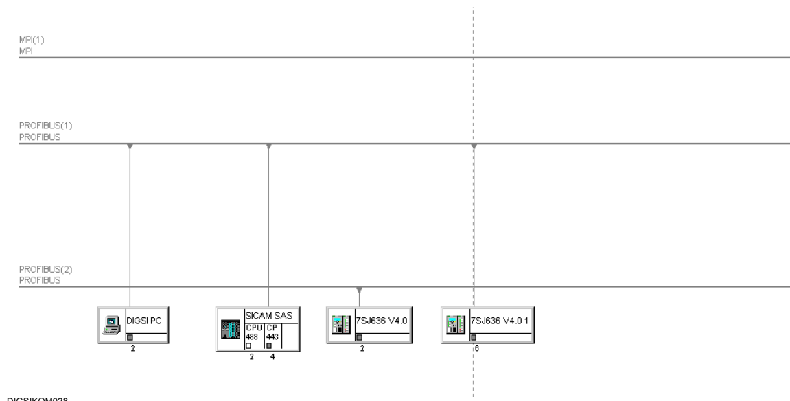
Рис. 7-35 Пример конфигурации сети с устройством SICAM и DIGSI ПК
