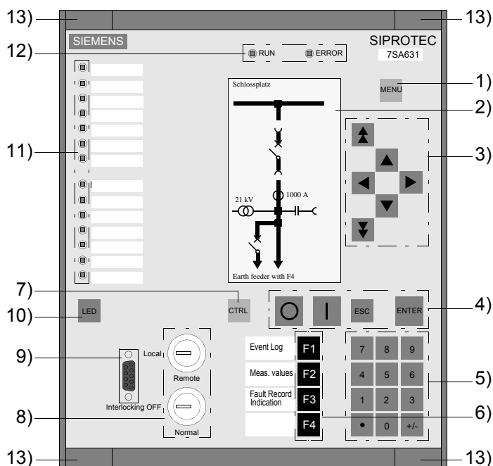
Рис. 2-2 Пример панели управления, вид спереди, размер корпуса 1/2
