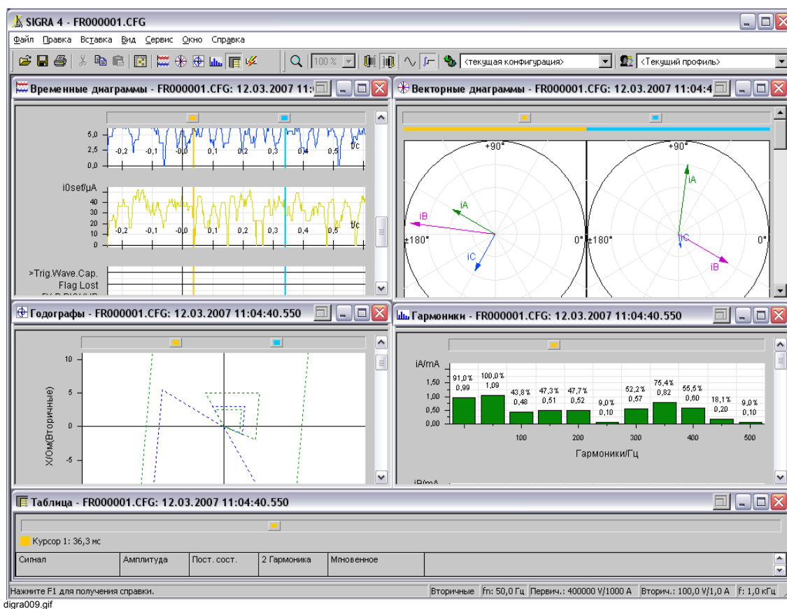
Рис. 6-31 SIGRA 4, Анализ осциллограмм повреждений, пример
