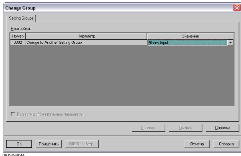
Рис. 5-6 Опция изменения группы уставок
