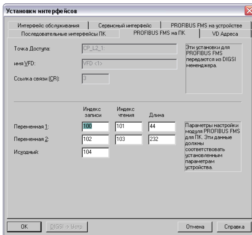
Рис. 7-37 Параметры интерфейса, закладка PROFIBUS FMS в ПК
