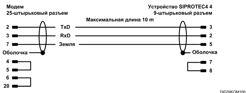
Рис. A-5 Электрическая схема для кабеля между модемом и устройством SIPROTEC 4
