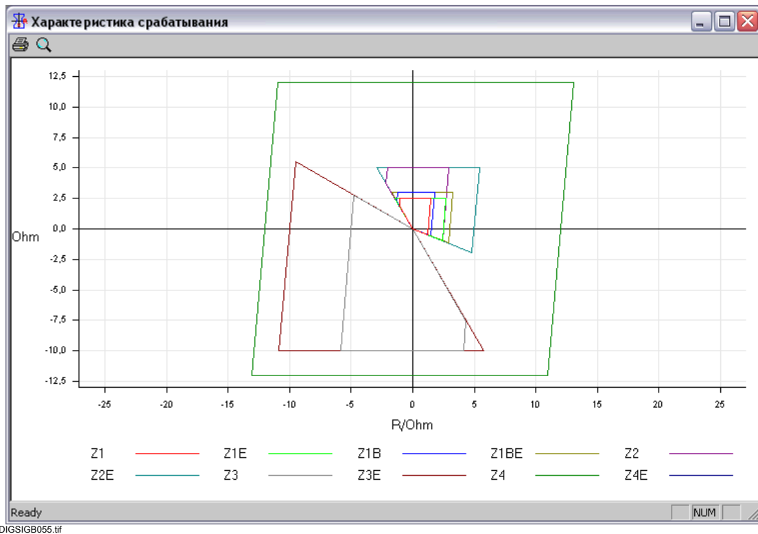
Рис. 5-86 Характеристики срабатывания
