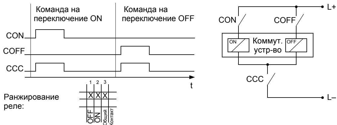
Рис. В-6 1 1/2-полюсная двойная команда
