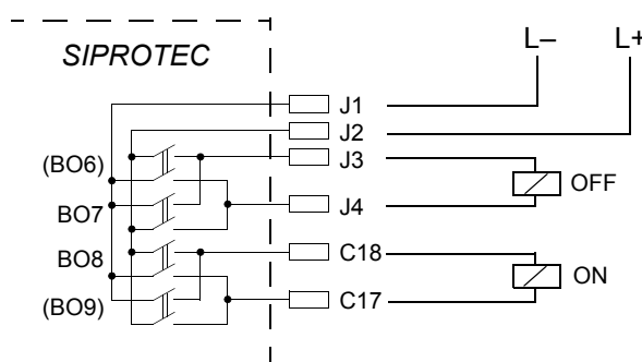
Рис. В-11 Фрагмент общей схемы вариантов с реле мощности BO6 - BO9 (например) и их цепи в соответствии с Рисунком В-12
