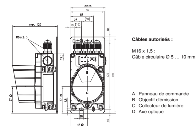
Figure 2.1 : Encombrement DDLS 200 avec câblage en cuivre
