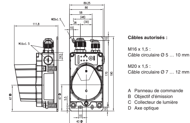
Figure 2.2 : Encombrement DDLS 200 avec câblage en fibre optique
