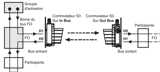
Figure 4.2: Raccordement du DDLS 200 à l'INTERBUS (conducteurs en fibre optique)
