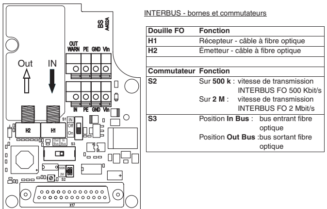
Figure 4.1: Platine des connexions variante INTERBUS
