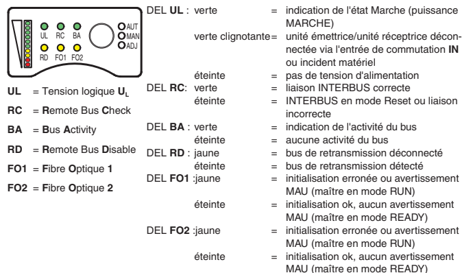
Figure 4.3: Éléments d'affichage / de commande variante INTERBUS
