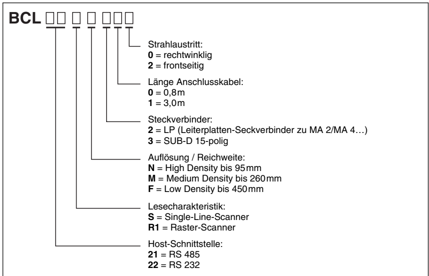
Bild 4.2: Typenschlüssel BCL 21/22
