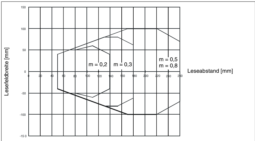
Bild 4.4: Lesefeld Optikausführung M (Medium Density, Normaler Bereich)
