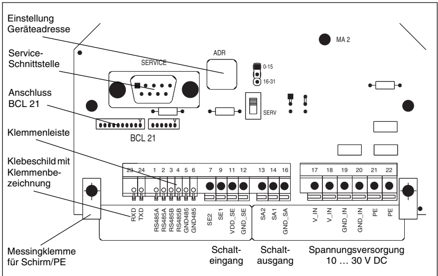
Bild 6.6: Anschlusseinheit MA 2
