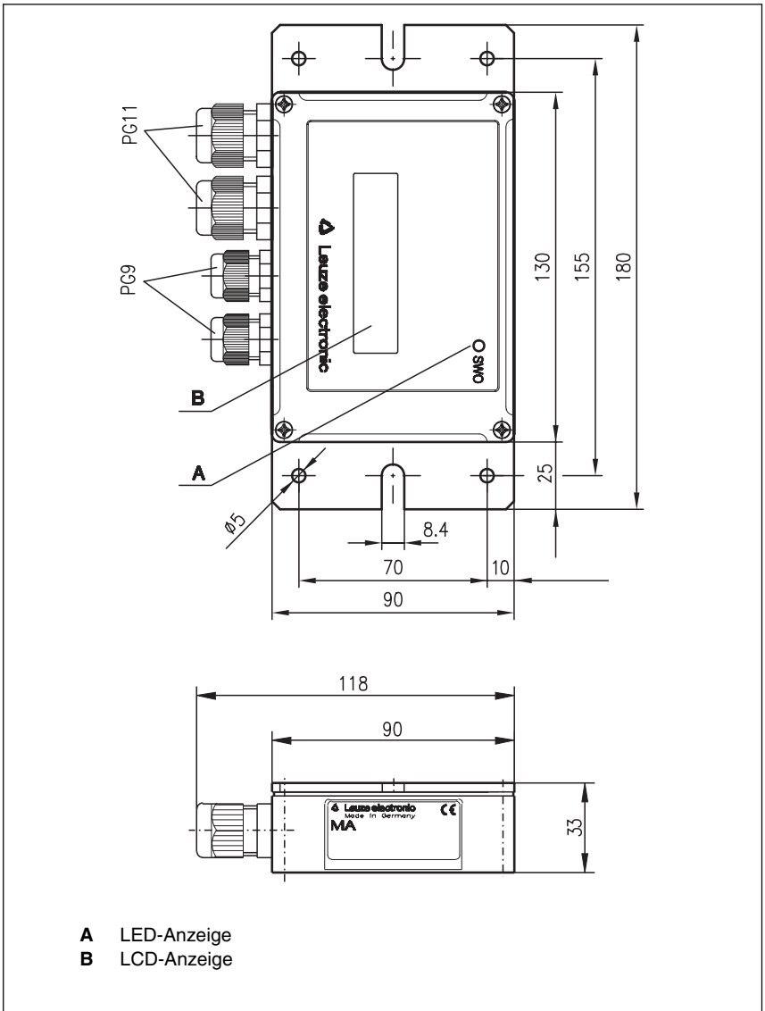
Bild 5.4: Maßzeichnung Anschlusseinheit MA 4/MA 4D
