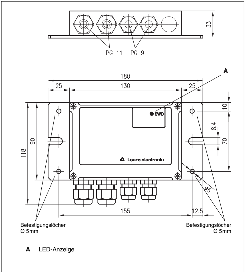
Bild 5.2: Maßzeichnung Anschlusseinheit MA 2
