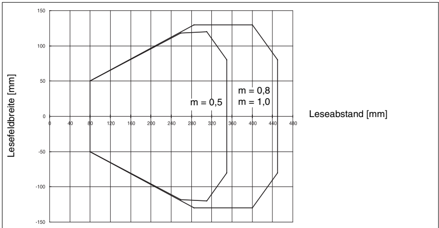
Bild 4.5: Lesefeld Optikausführung F (Low Density, Weiter Bereich)
