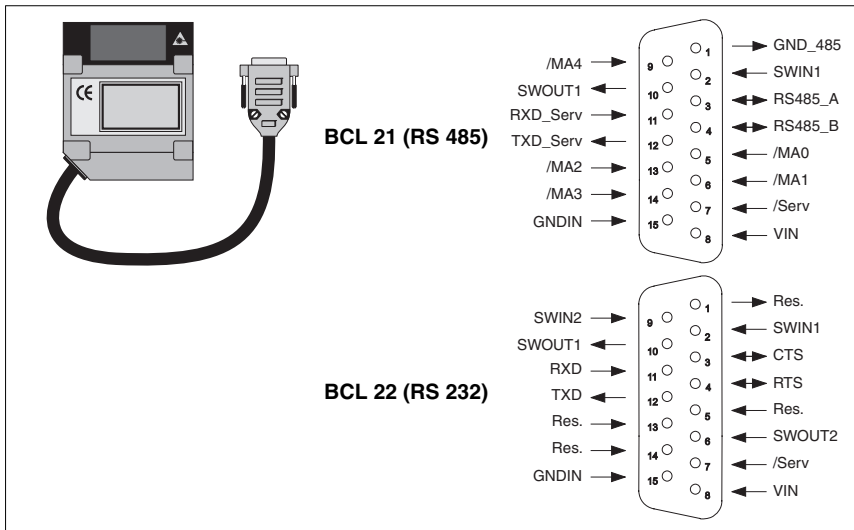
Bild 6.4: BCL 21/22 SUB-D-Steckerbelegung
