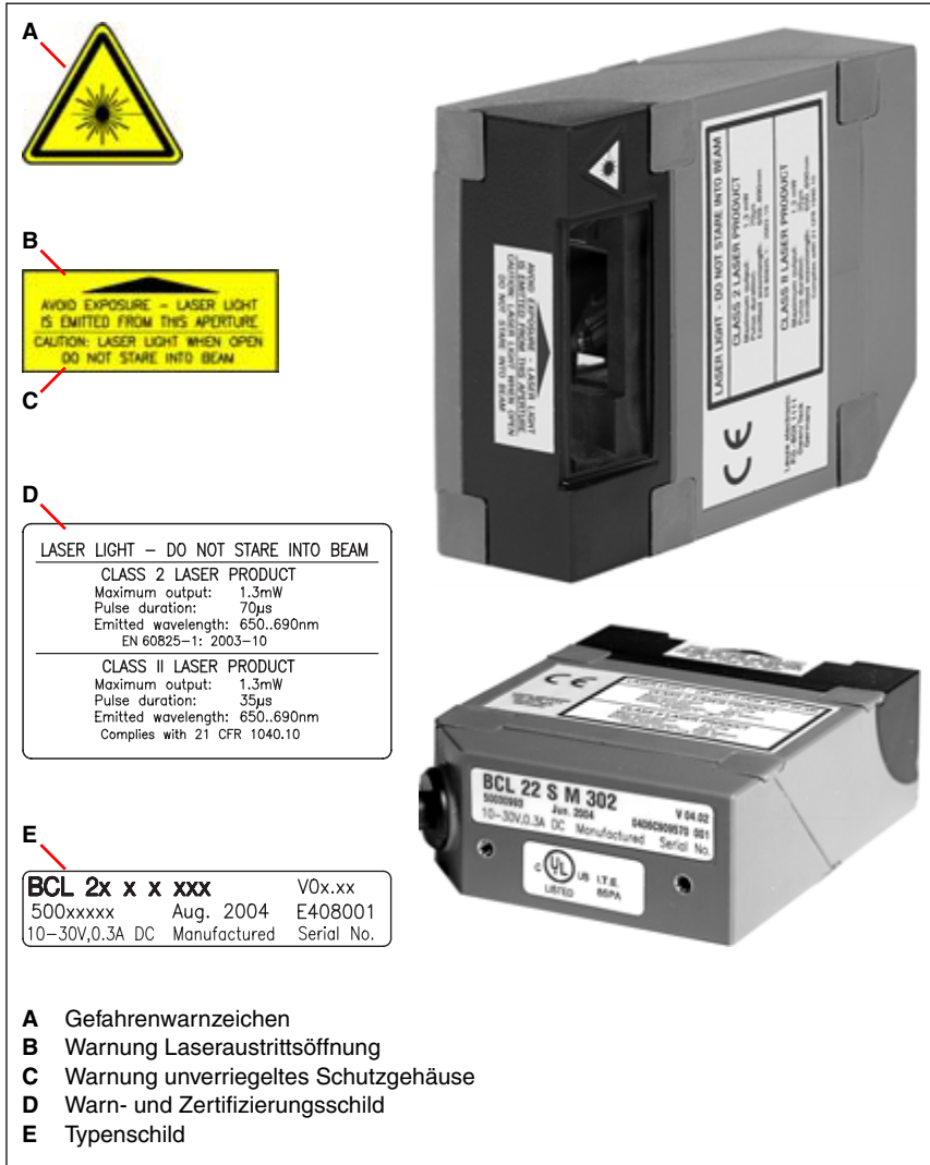
Bild 2.1: Anbringung der Aufkleber mit Warnhinweisen am BCL 21/22
