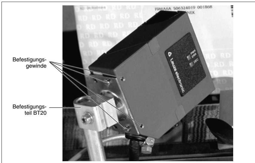
Bild 6.2: Befestigungsbeispiel BCL 21/22
