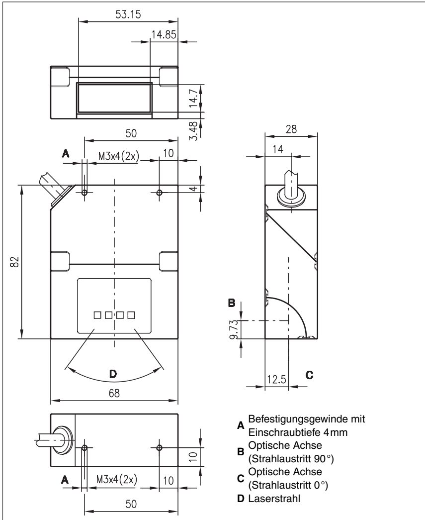
Bild 4.1: Maßzeichnung BCL 21/22
