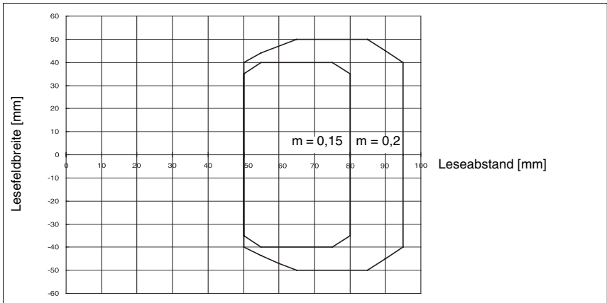
Bild 4.3: Lesefeld Optikausführung N (High Density)
