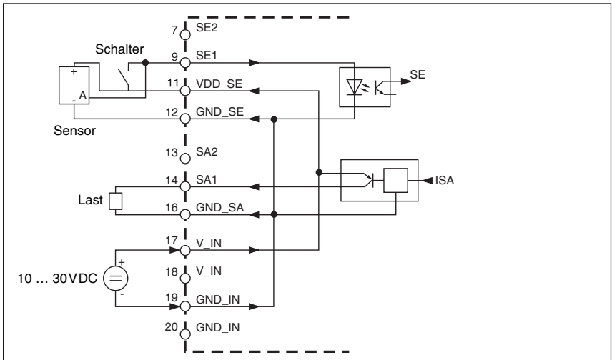
Bild 6.7: Beschaltung MA 2
