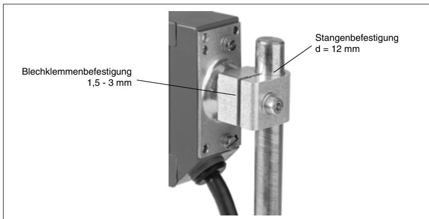
Bild 5.7: Befestigungsteil BT 20
