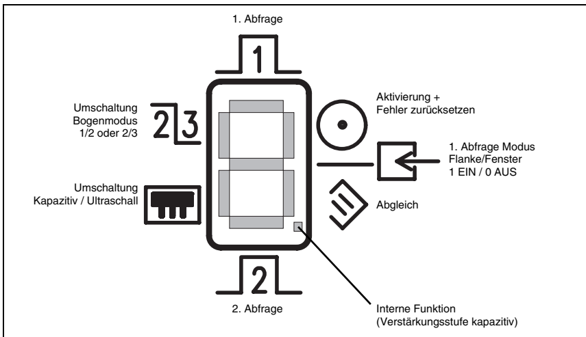
Bild 5.2: Steuereingänge
