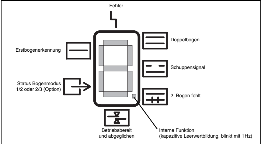
Bild 5.3: Steuerausgänge
