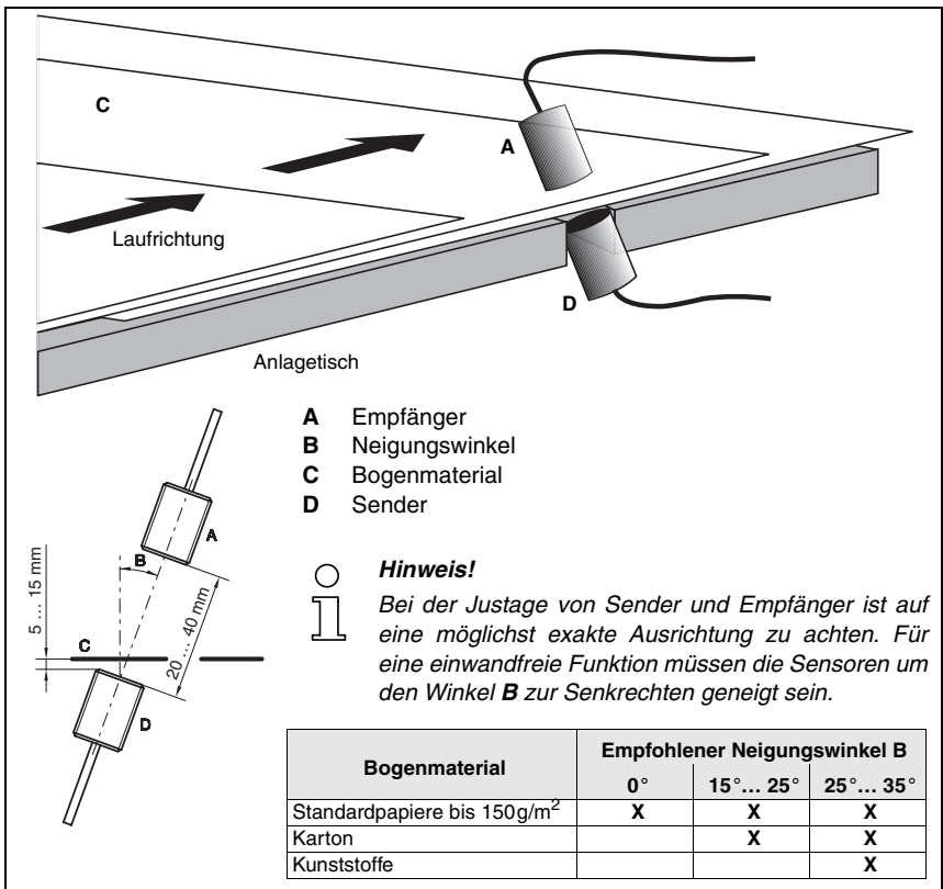
Bild 4.2: Montage der Ultraschall-Sensoren
