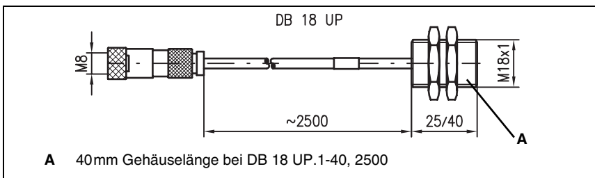
Bild 9.3: Ultraschallwandler DB 18 UP
