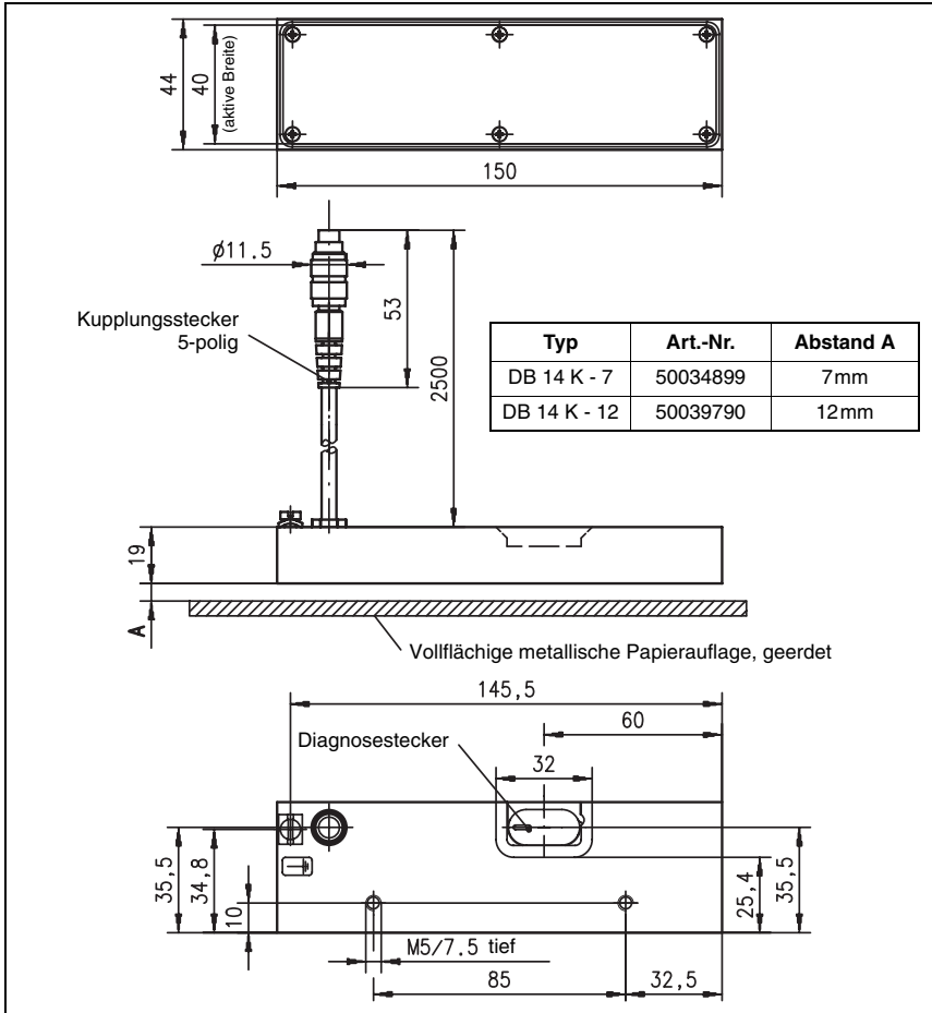
Bild 9.2: kapazitiver Sensor DB 14 K
