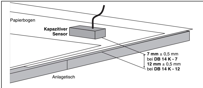
Bild 4.3: Montage des kapazitiven Sensors
