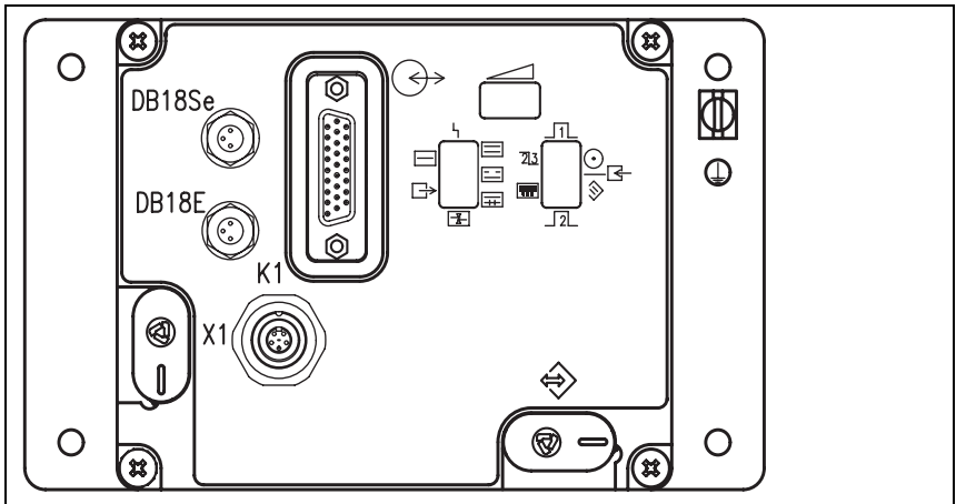
Bild 5.1: Auswerteeinheit VDB 14B
