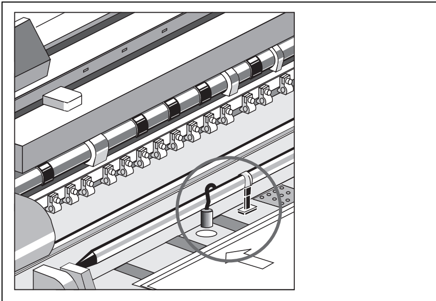
Bild 4.1: Beispiel für die Anordnung der Sensoren
