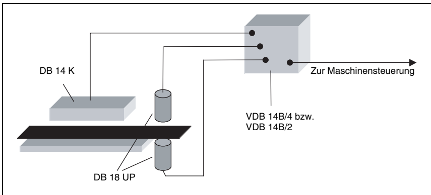
Bild 3.1: DB 14B Systemaufbau
