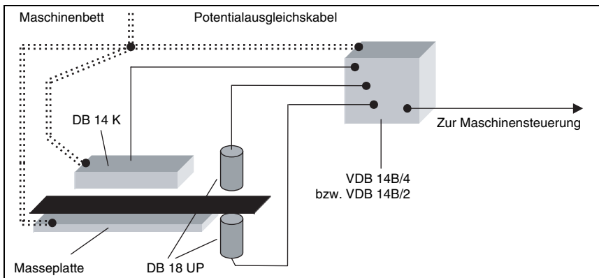
Bild 4.4: Potentialausgleich und Anschluss
