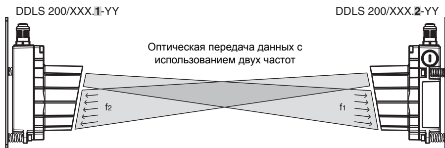
Рис. 1.1: Принцип действия
