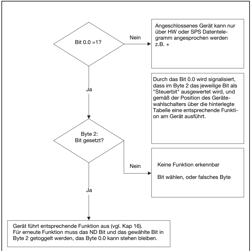
Bild 11.2: Befehlsausführung nach Aktivierung des Command Mode
