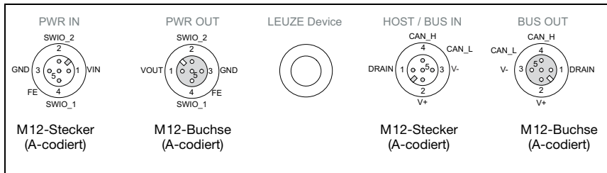
Bild 3.1: Anschlüsse der MA 235 i
