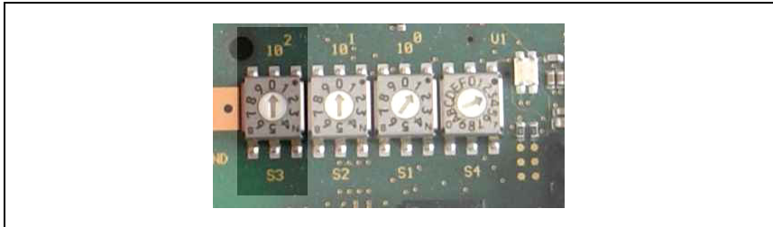
Bild 3.3: Drehschalter zur Baudrateneinstellung
