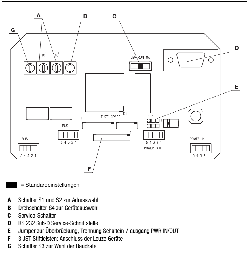
Bild 8.2: Vorderansicht: Bedienelemente der MA 235 i
