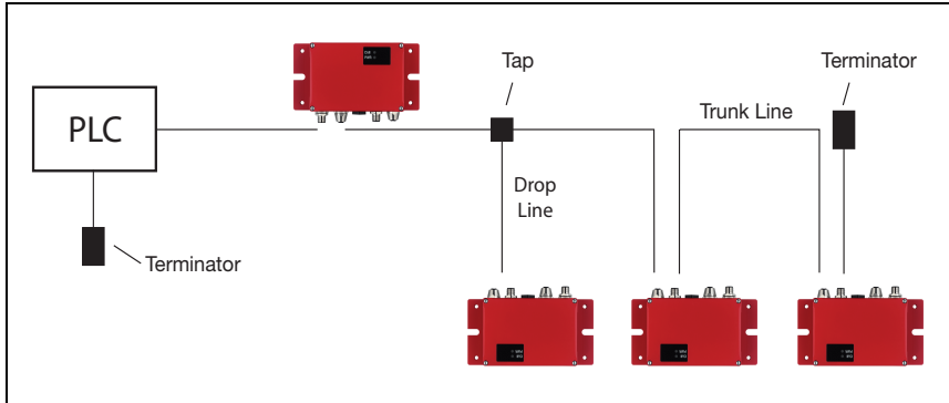
Bild 4.4: Bustopologie
