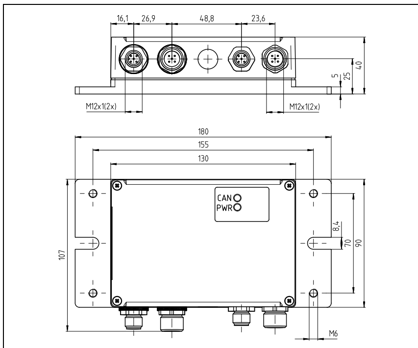
Bild 5.1: Maßzeichnung MA 235 i
