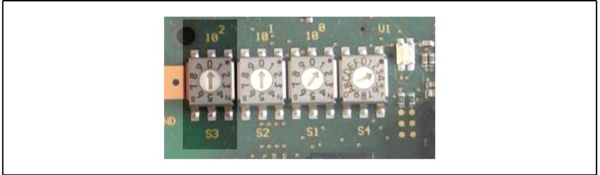
Bild 12.2: Drehschalter zur Baudrateneinstellung
