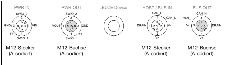
Bild 12.3: Anschlüsse der MA 235i von unten gesehen, Gerät auf Montageplatte
