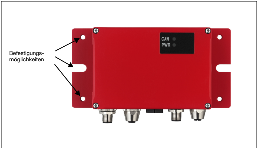
Bild 6.2: Befestigungsmöglichkeiten
