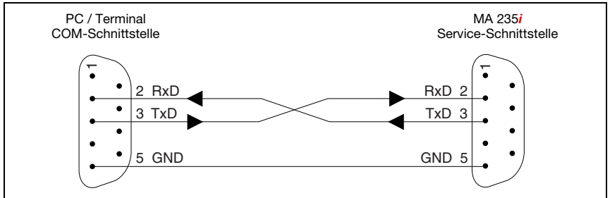
Bild 4.3: Verbindung der Service-Schnittstelle mit einem PC/Terminal
