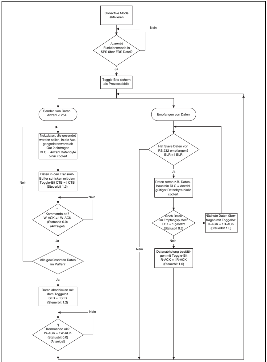
Bild 11.1: Schema der Datenübertragung mit langen Online-Kommandos
