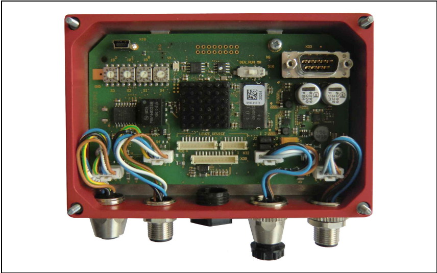
Bild 7.3: MA 235i offen
