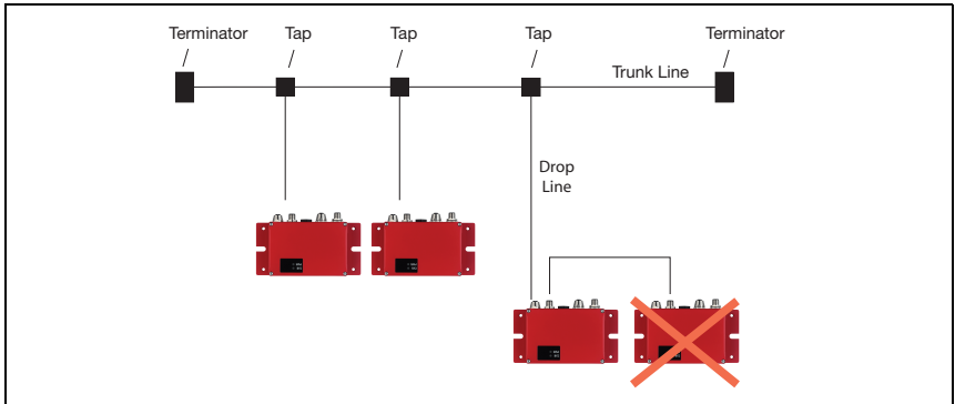
Bild 4.5: Unzulässige Vernetzung innerhalb einer Drop Line
