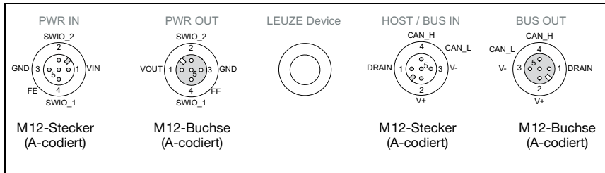
Bild 7.2: Anschlüsse der MA 235 i
