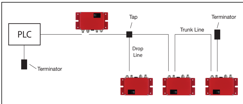
Figura 4.4: Topología de bus
