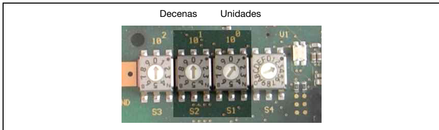
Figura 3.2: Interruptores giratorios para el ajuste de dirección
