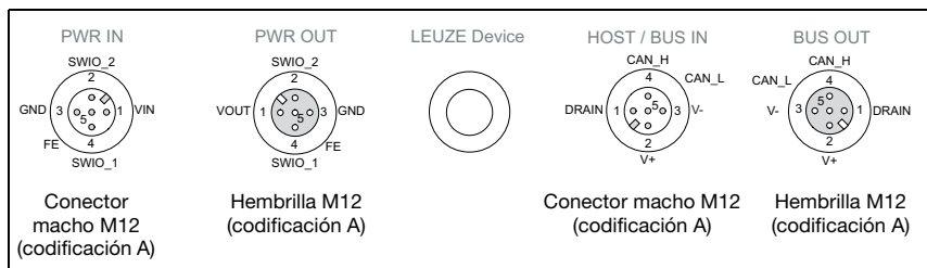
Figura 3.1: Conexiones de la MA 235i
