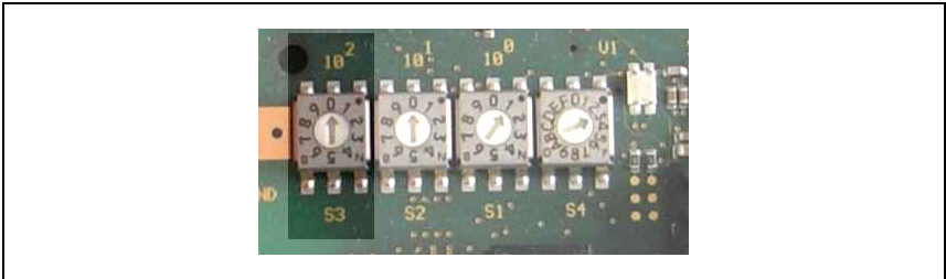
Figura 3.3: Interruptor giratorio para el ajuste de la velocidad de transmisión
