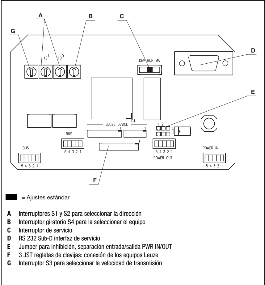
Figura 8.2: Vista frontal: elementos de mando de la MA 235 i
