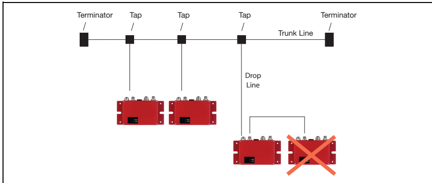
Figura 4.5: Interconexión no permitida dentro de un cable de derivación
