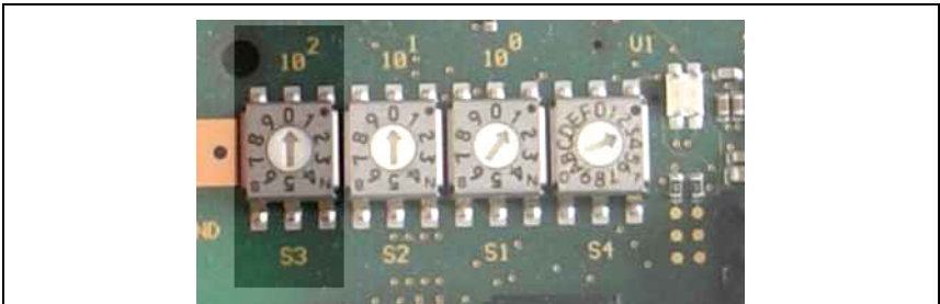
Figura 8.7: Interruptor giratorio para el ajuste de la velocidad de transmisión
