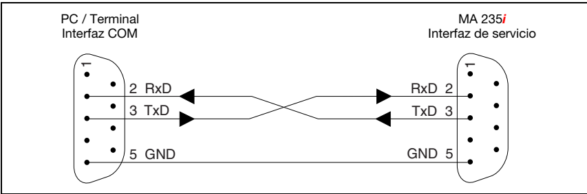
Figura 7.6: Conexión de la interfaz de servicio con un PC o terminal
