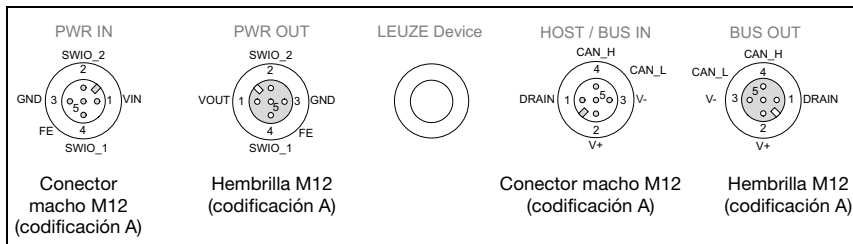
Figura 7.2: Conexiones de la MA 235 i
