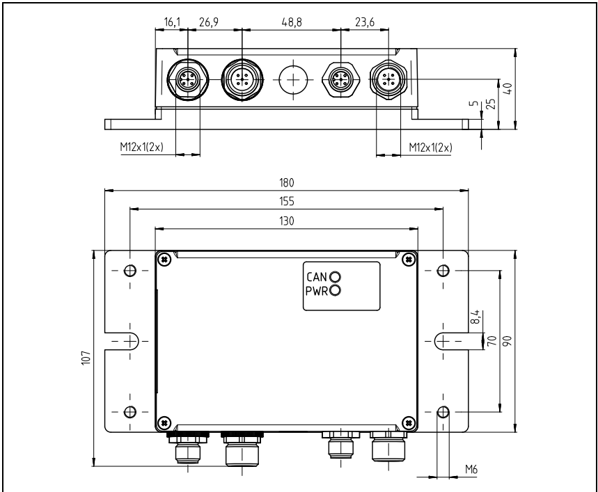
Figura 5.1: Dibujo acotado MA 235 i
