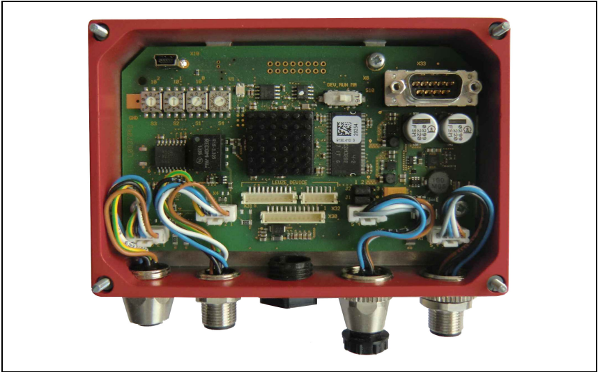
Figura 7.3: MA 235i abierta
