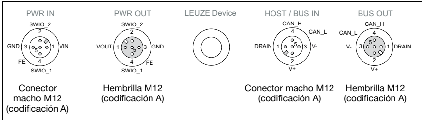
Figura 12.3: Conexiones de MA 235i vistas desde abajo, equipo sobre la placa de montaje
