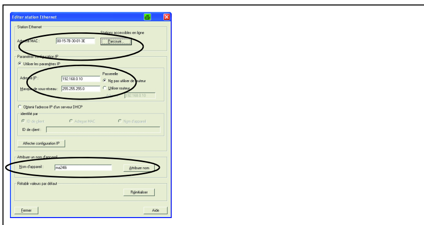
Figure 12.2 : Adresse MAC - adresse IP - nom d'appareil individuel
