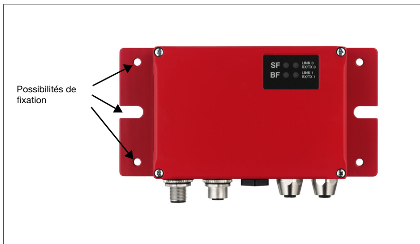
Figure 6.2 : Possibilités de fixation
