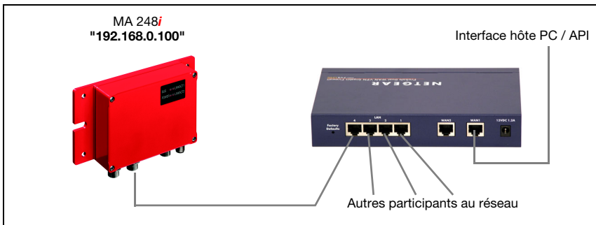
Figure 4.4 : PROFINET-IO avec topologie en étoile
