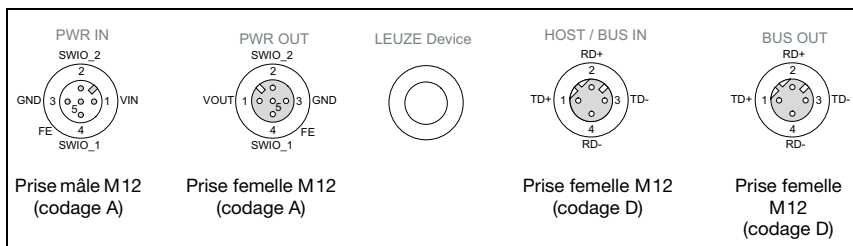
Figure 7.2 : Raccordements de la MA 248 i
