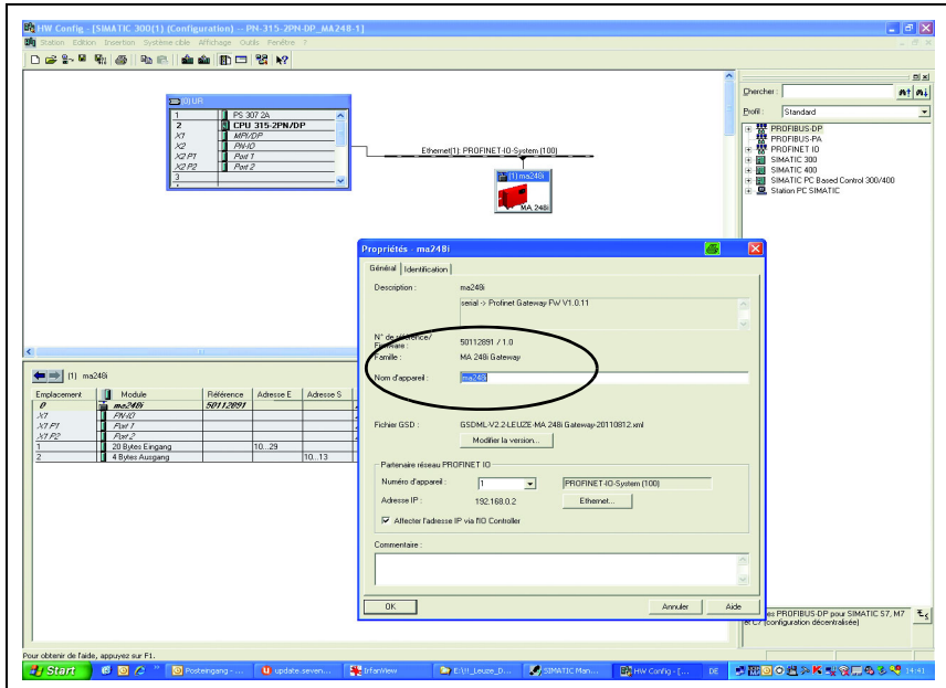
Figure 12.1 : Attribution des noms d'appareil à des adresses IP
