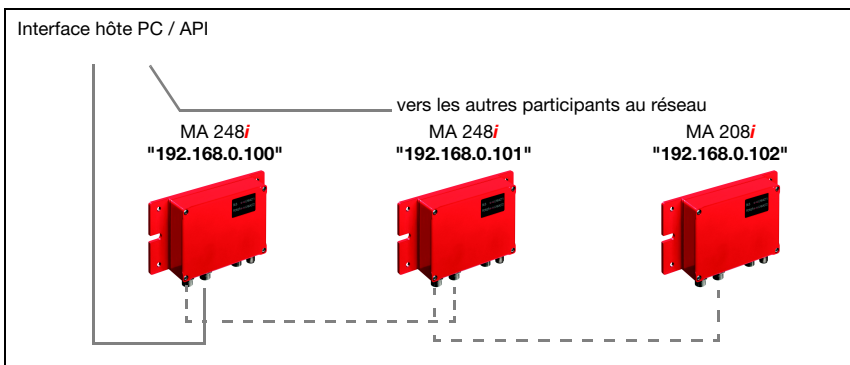
Figure 4.5 : PROFINET-IO avec topologie en bus
