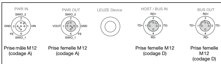
Figure 12.1 : Raccordements de la MA 248 i , vue de dessous, appareil sur une plaque de montage
