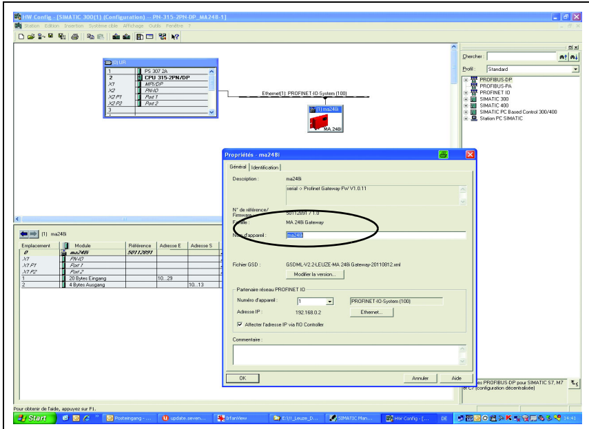
Figure 3.2 : Attribution des noms d'appareil à des adresses IP
