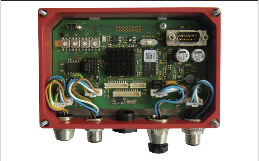
Figure 7.4 : MA 248 i ouverte
