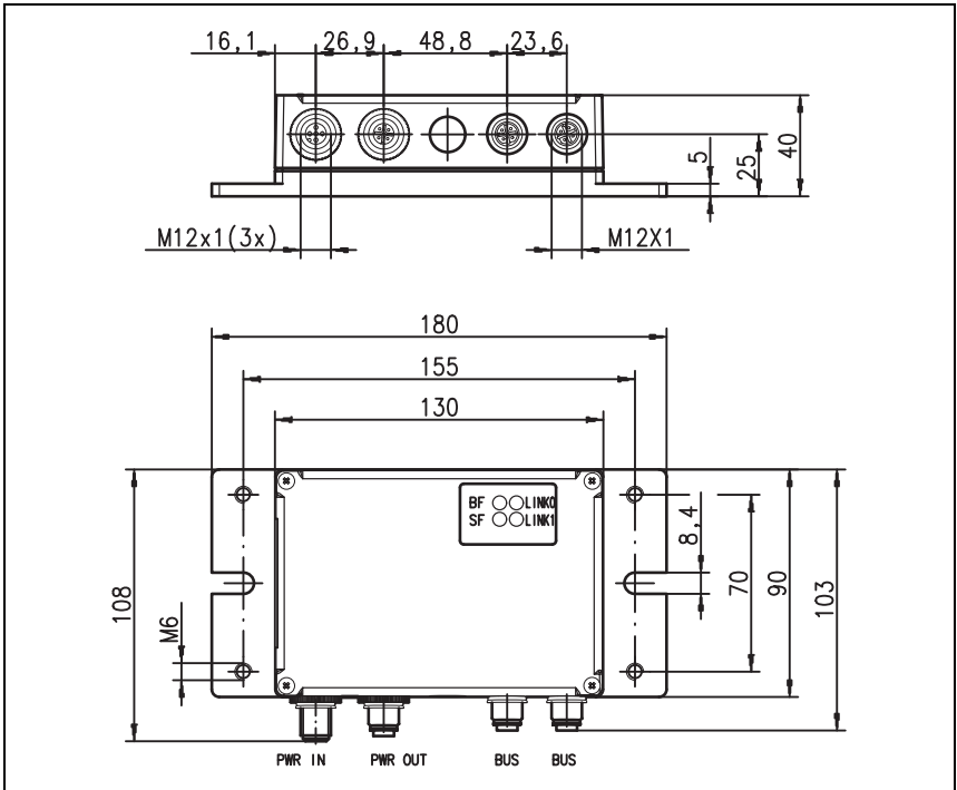
Figure 5.1 : Encombrement de la MA 248 i
