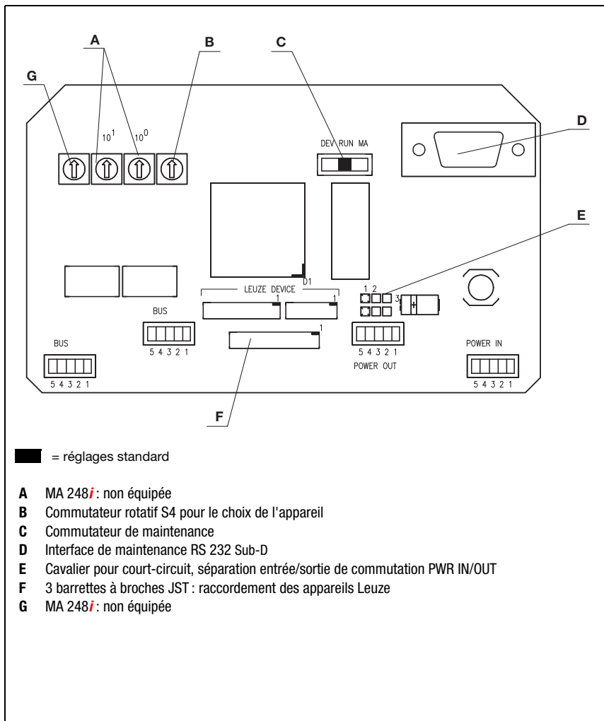
Figure 8.2 : Vue de face : éléments de commande de la MA 248 i
