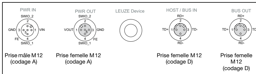
Figure 3.1 : Raccordements de la MA 248 i
