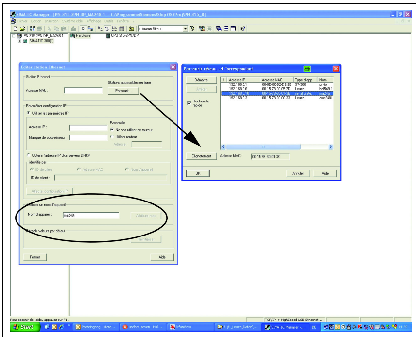
Figure 12.1 : Affectation des noms d'appareil aux appareils IO configurés
