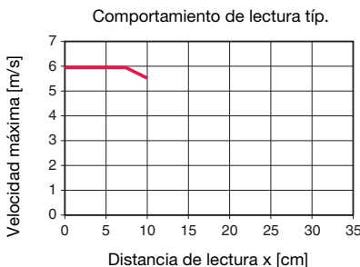
Figura 3.2: Comportamiento de lectura típico - Unidad de inscripción-lectura RFM 32
