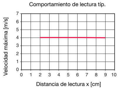
Figura 3.3: Comportamiento de lectura típico - unidad de lectura/escritura RFM 32 Ex n
