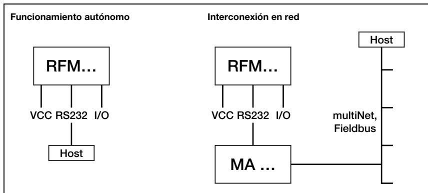
Figura 3.9: Conexión autónoma / interconexión en red
