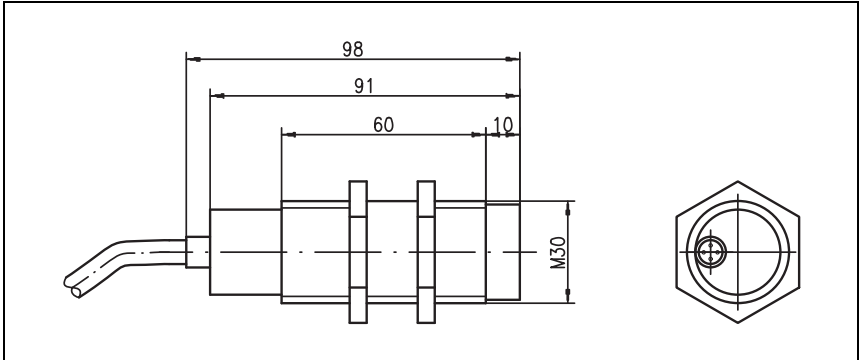
Figura 4.1: Dibujo acotado del equipo de lectura/escritura RFM 12 SL 200
