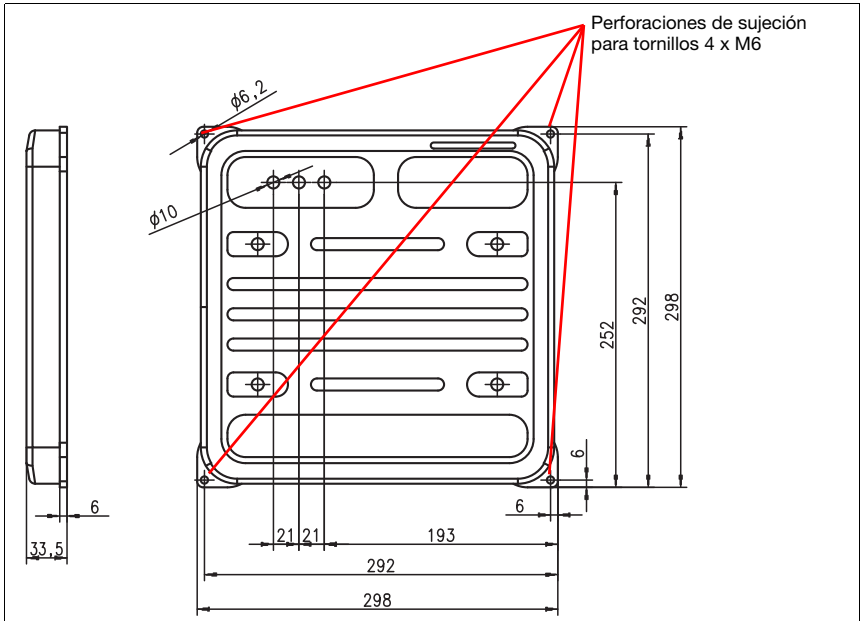
Figura 5.3: Perforaciones de sujeción RFM 62
