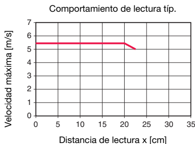
Figura 3.4: Comportamiento de lectura típico - Unidad de inscripción-lectura RFM 62
