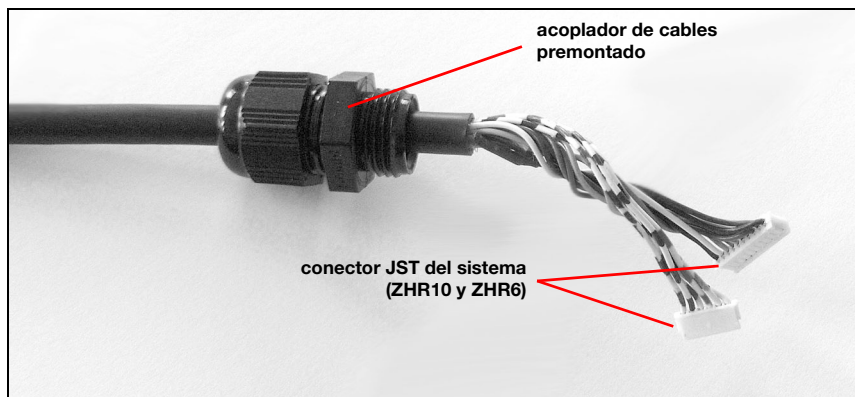
Figura 6.1: Conexión eléctrica con cable de conexión preconfeccionado
