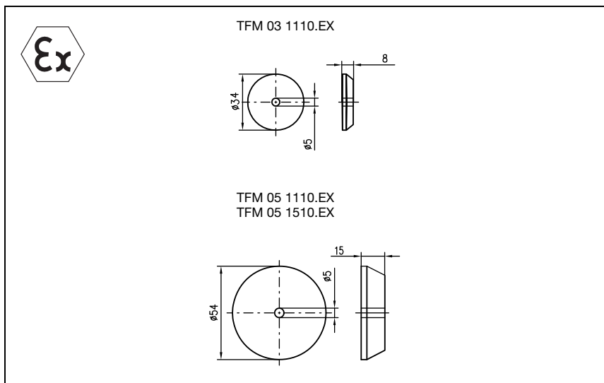
Figura 4.6: Dibujo acotado del transponder Ex TFM 0x 1x10.EX
