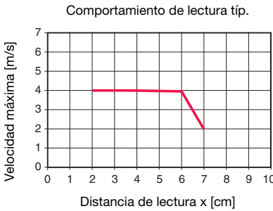
Figura 3.3: Comportamiento de lectura típico - unidad de lectura/escritura RFM 32 Ex n
