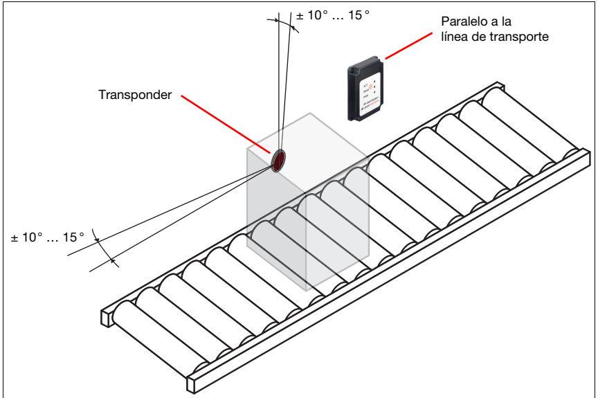
Figura 5.4: Disposición de los equipos de lectura/escritura en la línea de transporte
