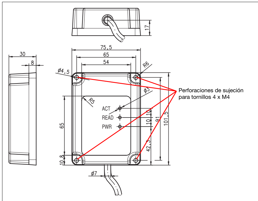
Figura 5.2: Perforaciones de sujeción RFM 32
