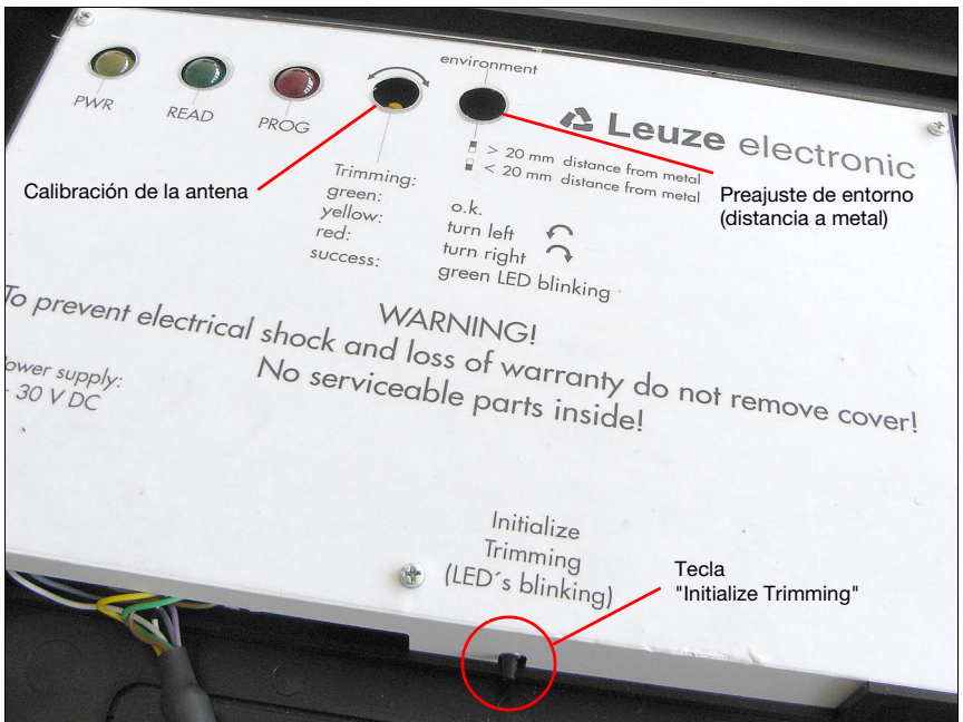
Figura 7.1: Calibración de la antena del RFM 62
