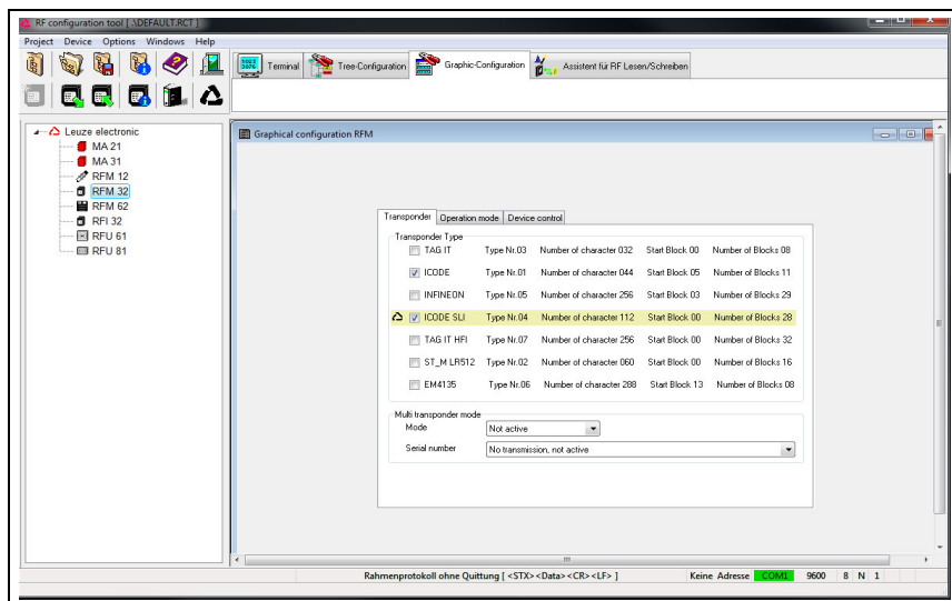
Figura 7.2: RF-Config – Ficha Transponder
