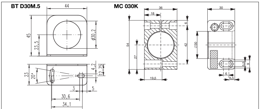
Figura 5.1: Sujeción del RFM 12 con accesorios de sujeción opcionales
