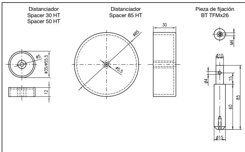
Figura 4.4: Dibujo acotado de distanciadores/piezas de sujeción para transponders
