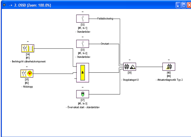
Fig 4.6: Exempel 1 Konfiguration av diagnosbyggstenen hos den säkra utgångsslav
