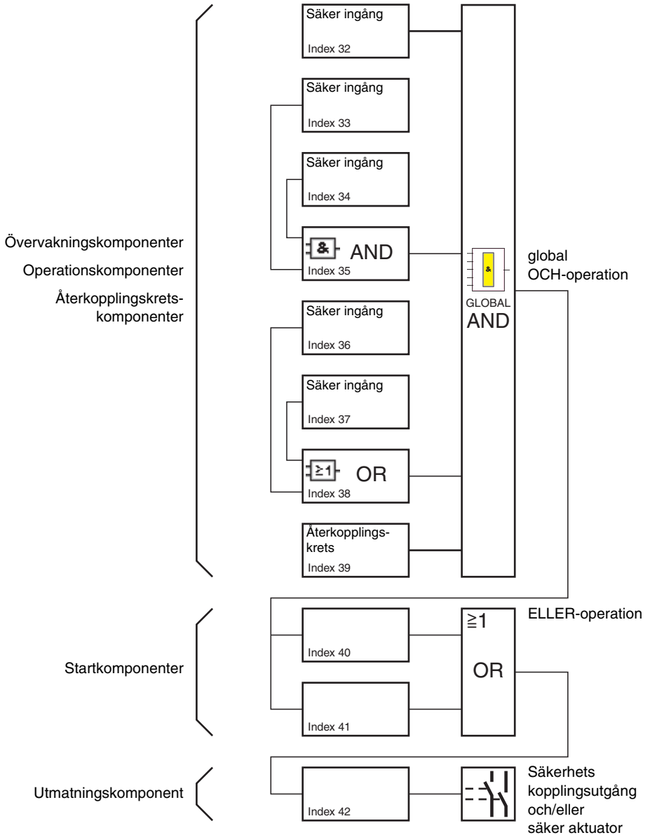
Fig 4.1: Rutin för utvärdering av de konfigurerade komponenterna
