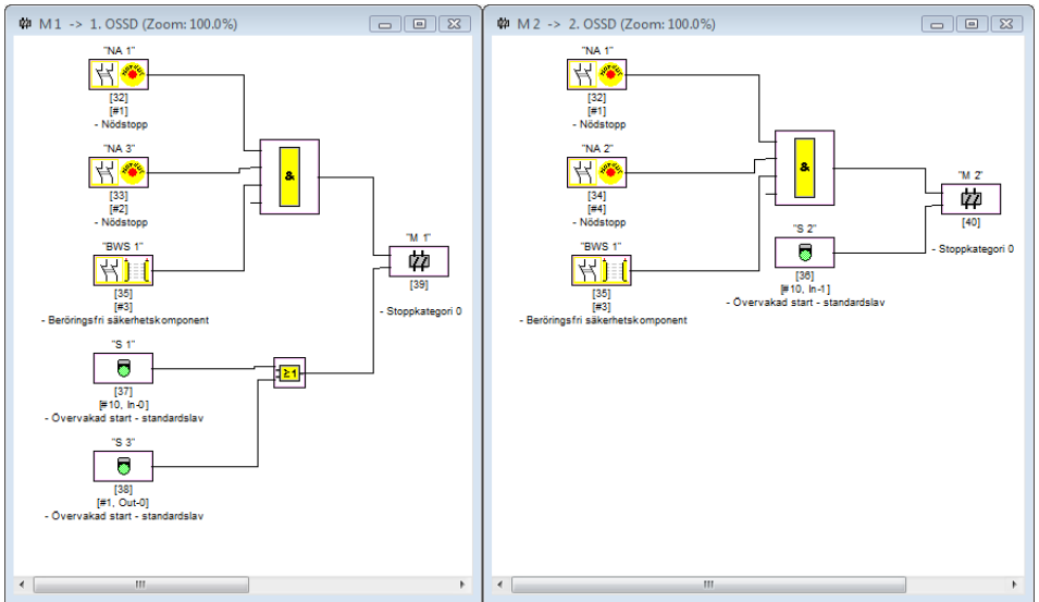
Fig 4.3: Exempel: En konfigureringsstruktur
