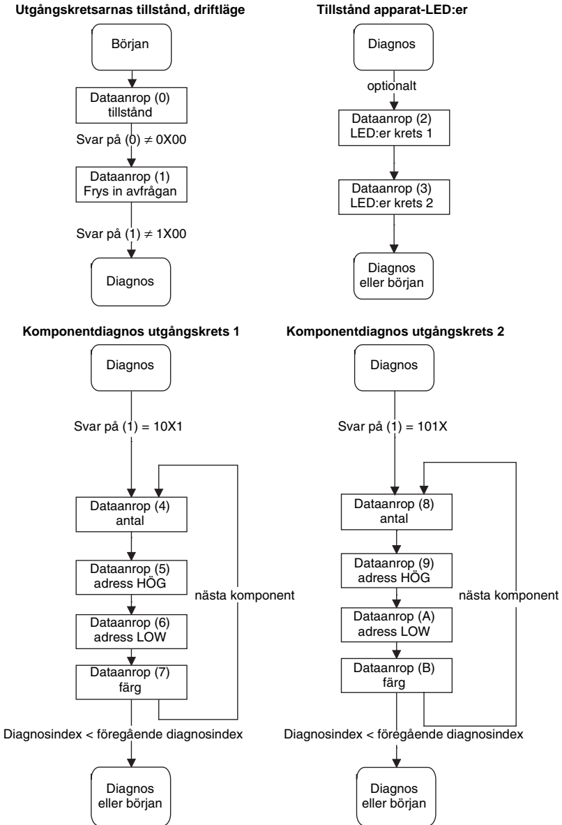
Fig 7.1: Avfrågningsprincip vid diagnos med sortering efter utgångskrets
