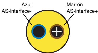
Cable redondo AS-interface (recomendado: cable flexible de energía H05VV-F2x1,5 según DIN VDE 0281)
