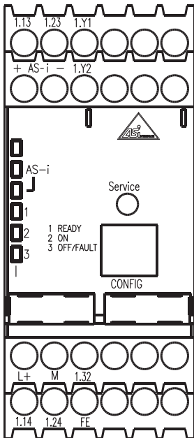
Figura 5.1: Disposición de los bornes / esquema de bloques para el monitor de seguridad AS-interface ASM1/1 y ASM1E/1
