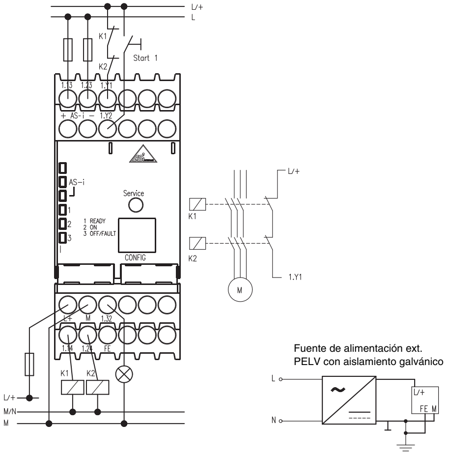
Figura 5.2: Sinopsis de las conexiones para el monitor de seguridad AS-interface ASM1/1 y ASM1E/1
