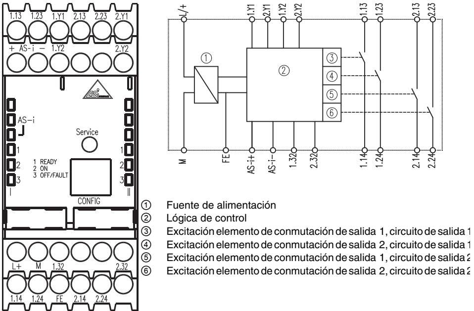
Figura 6.1: Disposición de los bornes / esquema de bloques para el monitor de seguridad AS-interface ASM1/2 y ASM1E/2
