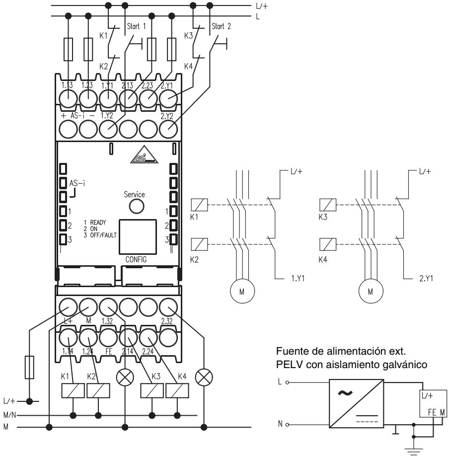
Figura 6.2: Sinopsis de las conexiones para el monitor de seguridad AS-interface ASM1/2 y ASM1E/2
