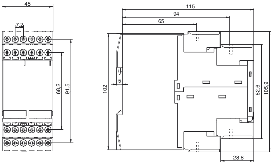
Figura 3.4: Dimensiones
