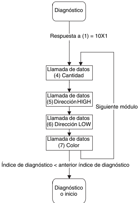
Figura 12.1: Principio de la consulta con circuitos de salida de diagnóstico clasificado
