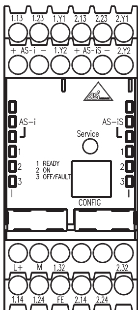
Figura 7.1: Disposición de los bornes / esquema de bloques para el monitor de seguridad AS-interface ASM2E/1 y ASM2E/2
