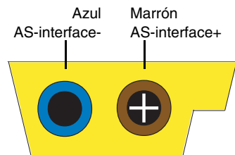
Cable plano AS-interface amarillo
