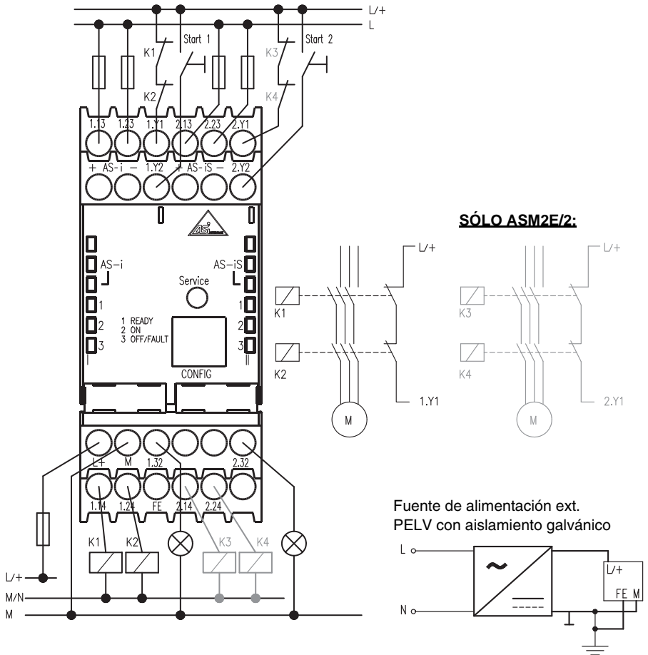
Figura 7.2: Sinopsis de las conexiones para el monitor de seguridad AS-interface ASM2E/1 y ASM2E/2
