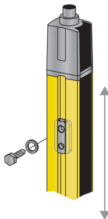
Figura 6.7: Montaje mediante tuercas correderas BT-NC60
