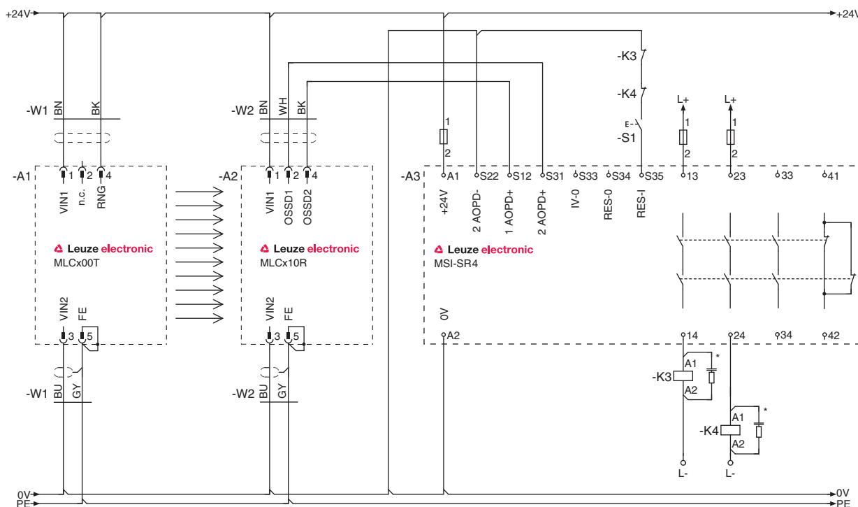
Figura 7.6: Ejemplo de circuito con módulo de seguridad posconectado MSI-SR4
