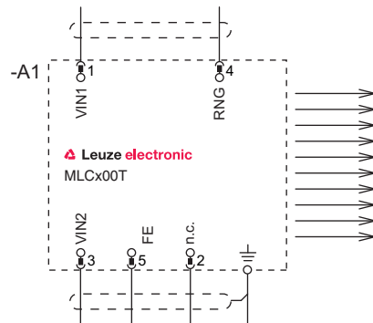
그림 7.2: 송신기 연결도
