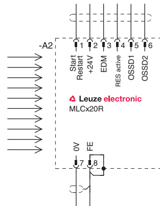
Figura 7.5: Esquema de conexión del receptor
