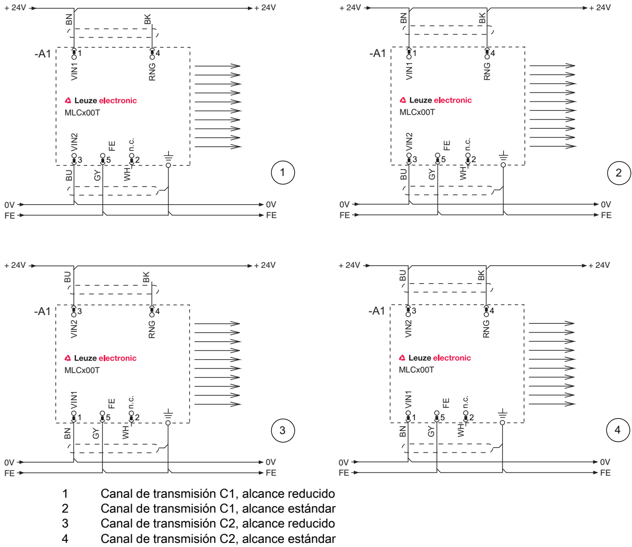
Figura 7.3: Ejemplos de conexión del emisor
