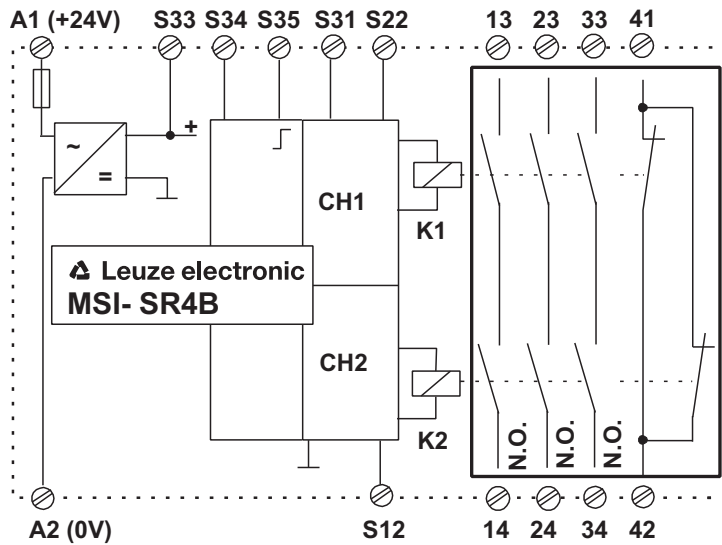
Bild 3.3: Innenschaltbild MSI-SR4B
