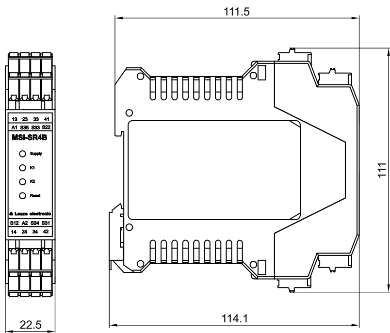
Bild 13.2: Maße MSI-SR4B-02
