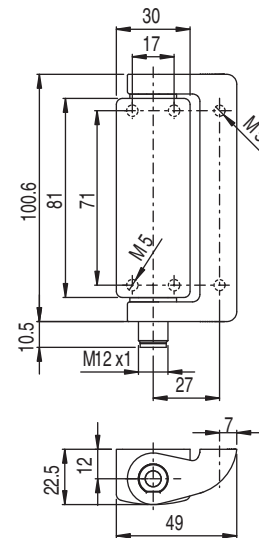
Bild 13.2: Maße S400-M4M12-B in mm
